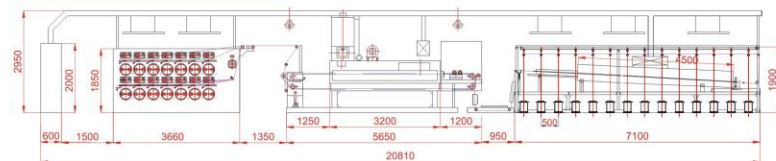
H3200-28-8平面布置图LAYOUT
