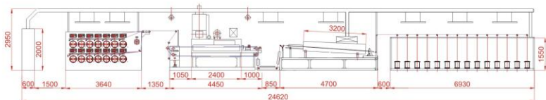
H2400-28-8平面布置图 LAYOUT
